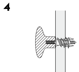
フック本体裏面が壁面に触れるまで しっかりとねじ込んで設置完了です。
