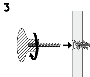
フック本体を回し、アンカーに合わせて ネジをねじ込みます。
